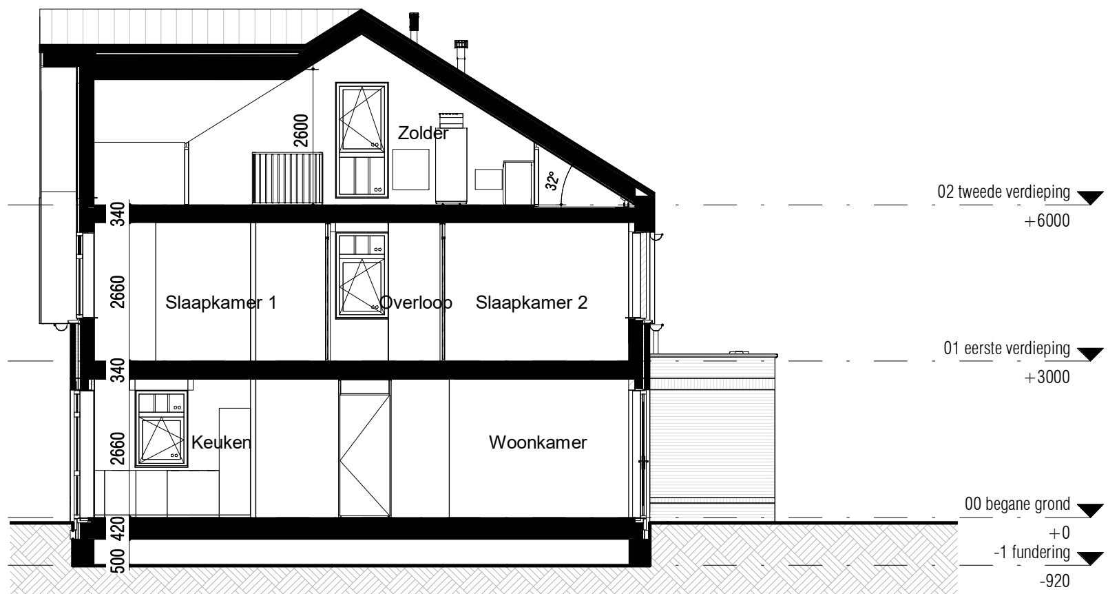
Doorsnede
