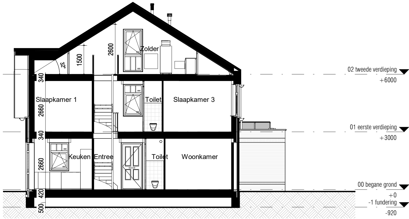
Doorsnede
