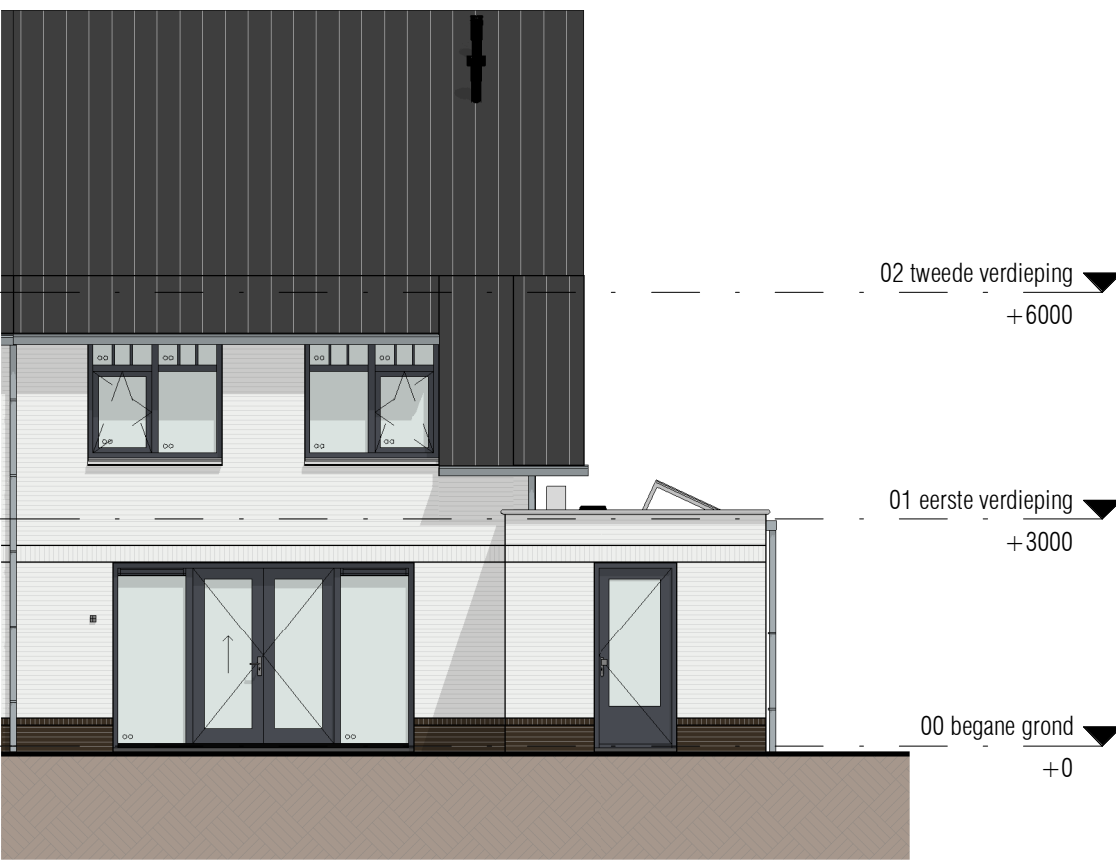
Achtergevel
