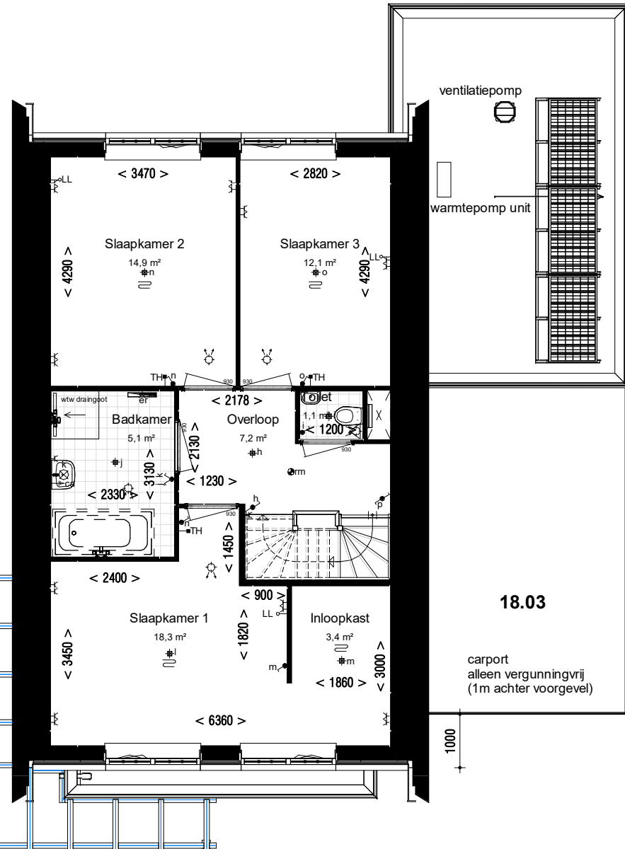
Eerste verdieping, 3000+P
