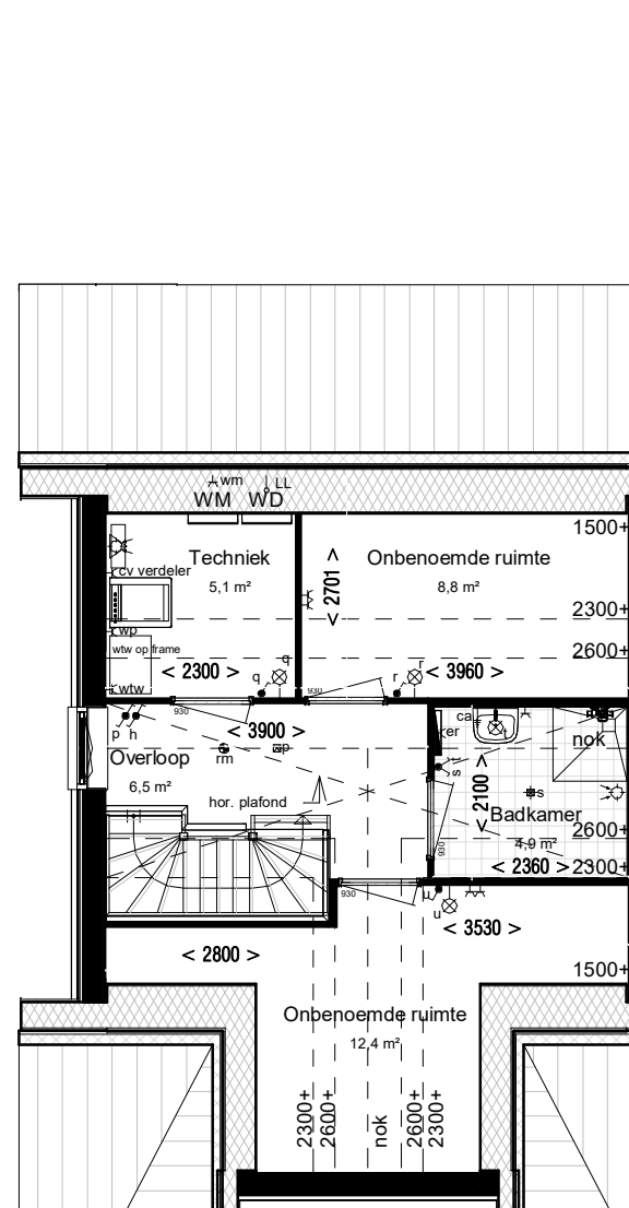
18.07 indeling tweede verdieping type 1
