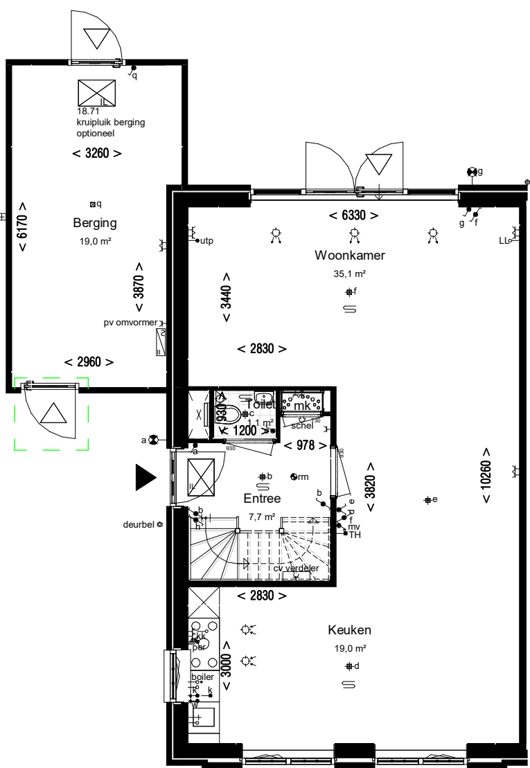
30.06 loopdeur i.p.v. kanteldeur naar de berging
