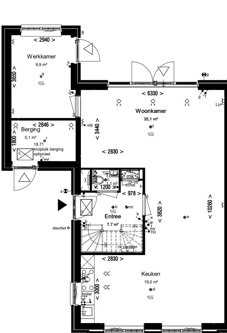
18.05a werkkamer in berging
