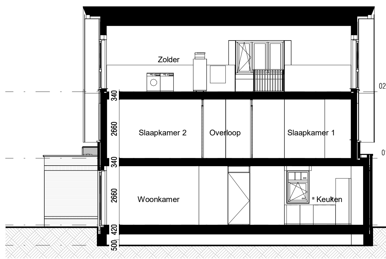
Doorsnede
